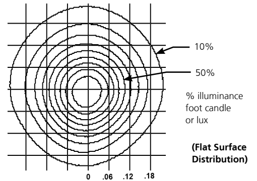
Iso-Illuminance Diagram
