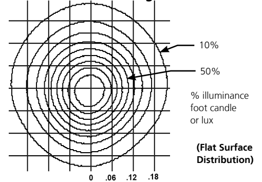
Iso-Illuminance Diagram
