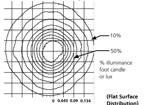
Iso-Illuminance Diagram
