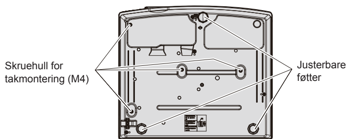
Skrueshullenes posisjoner for takmontering og justerbare føtter
